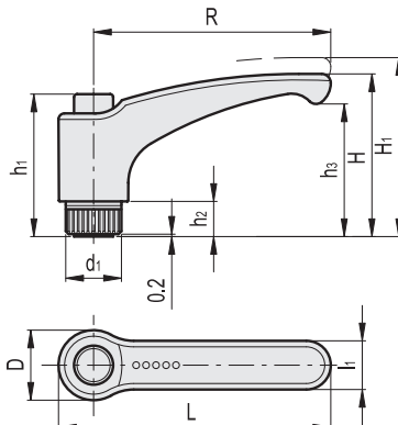
ERX-B
